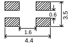
Land Pattern(mm)
