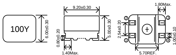
Dimensions外形尺寸(mm)
