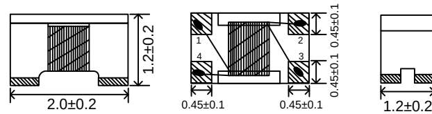
Dimensions外形尺寸(mm)
