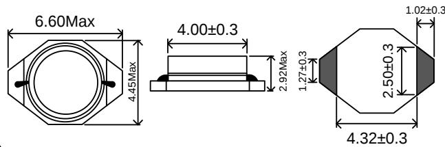
Dimensions外形尺寸(mm)
