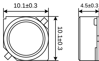
Dimensions外形尺寸(mm)
