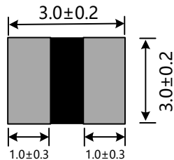
Dimensions外形尺寸(mm)
